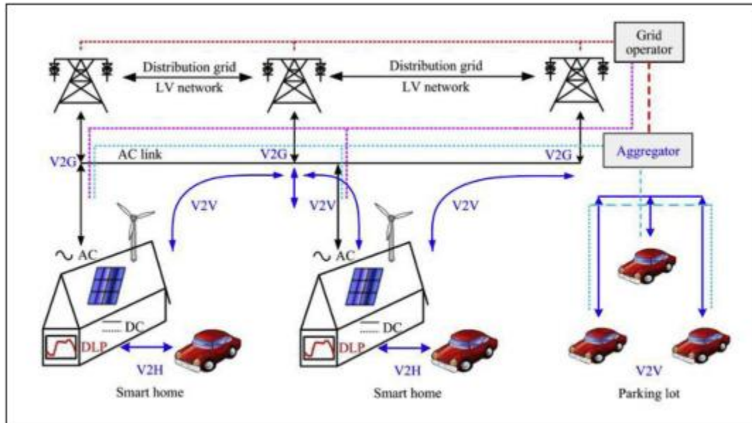
Fig: 3 Bi-directional EV settings (V2G, V2V y V2H).
