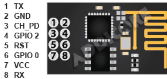
Fig6. Wifi Module
