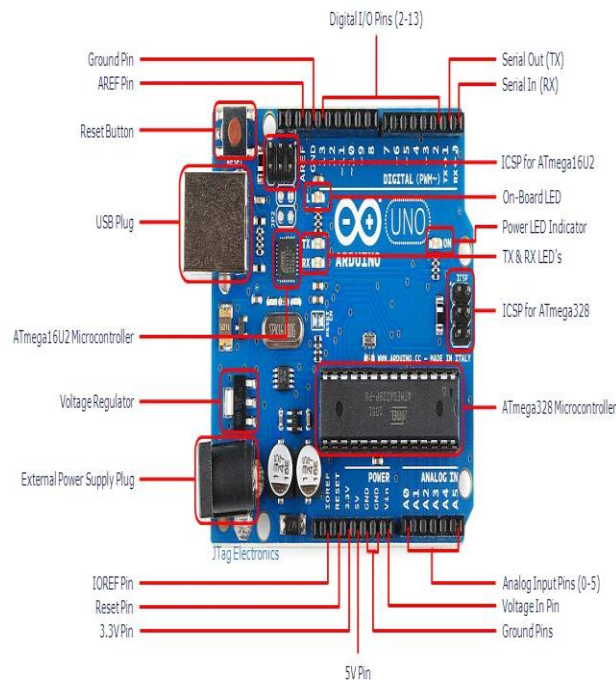
Fig2. Arduino Uno Board
